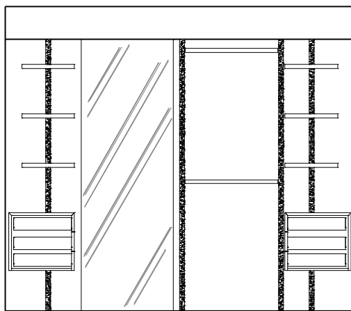
Ansicht B
